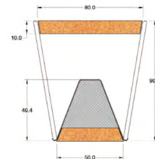
Sección
