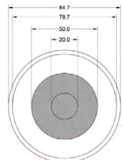
Planta
